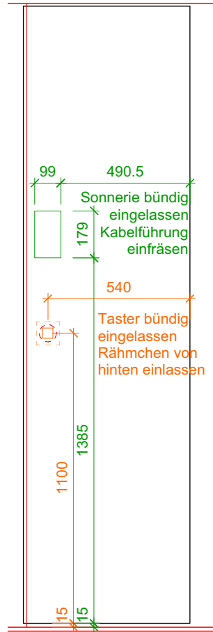
D-D
